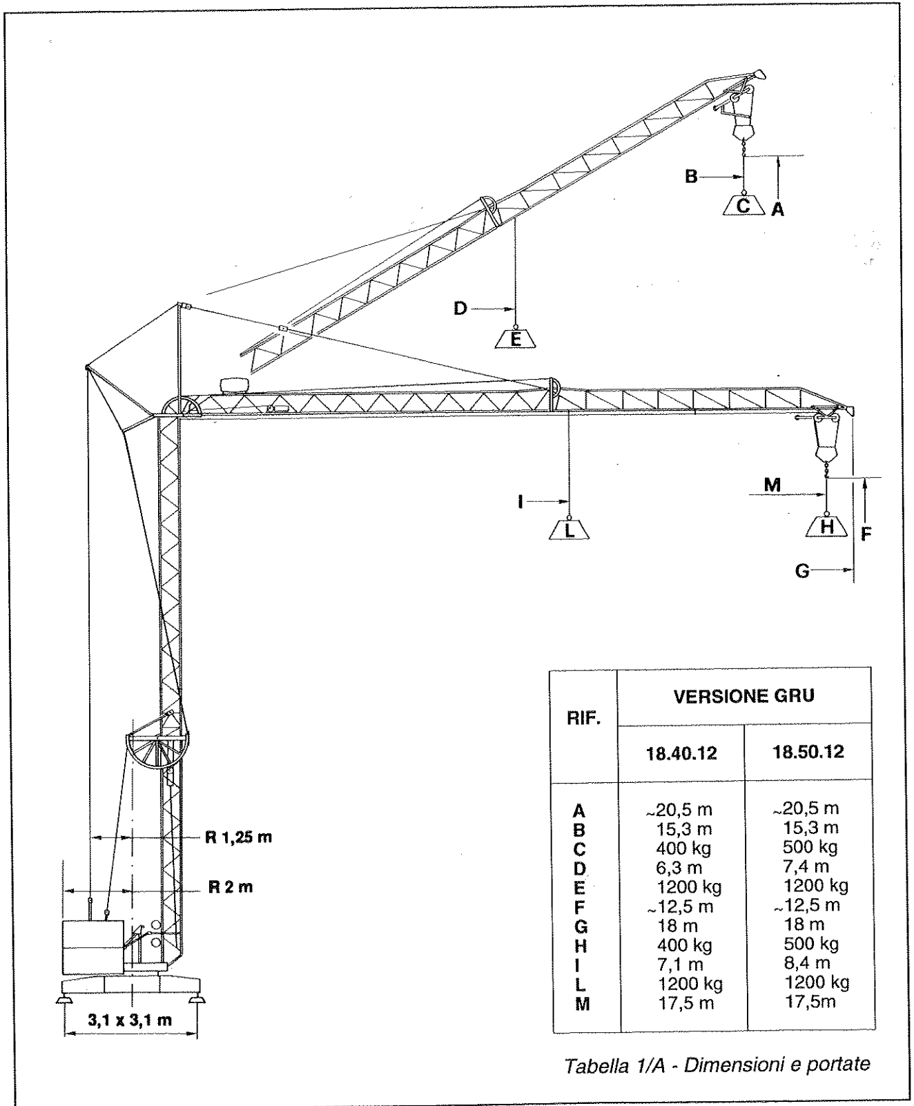
Fig. 1 - Braccio da 18 metri
